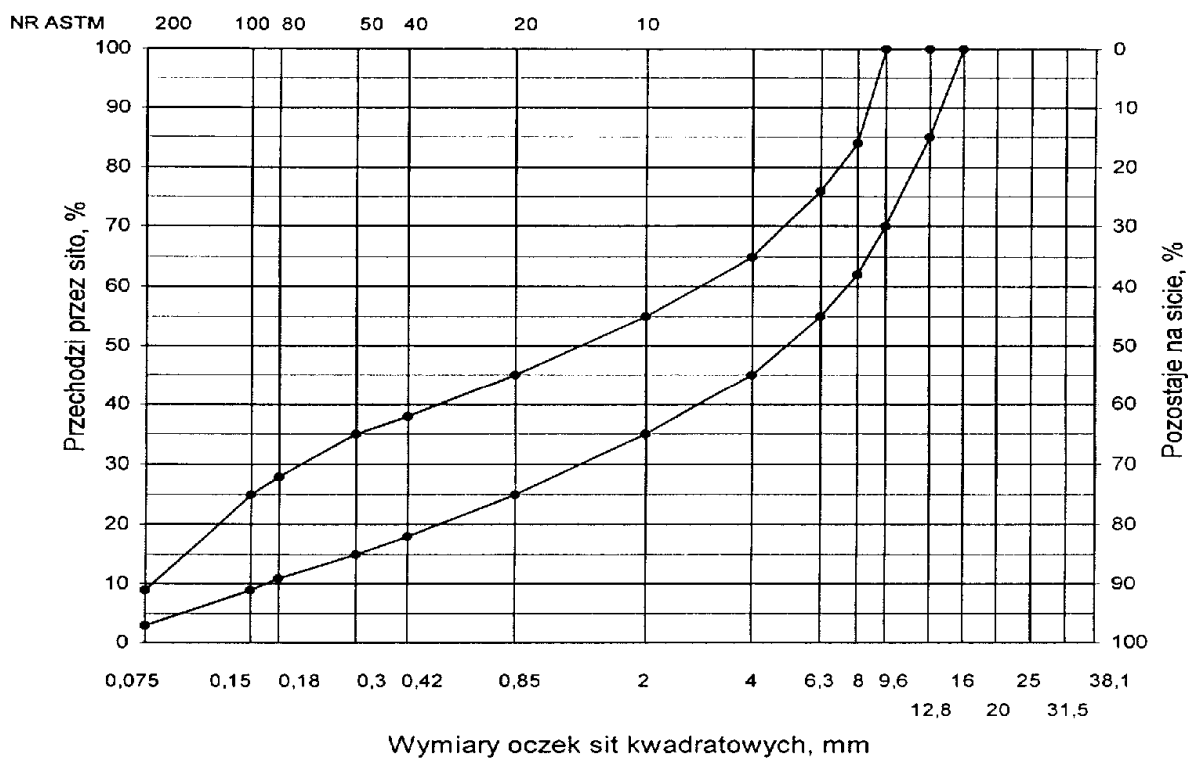
Rys. 2. Krzywe graniczne uziarnienia mieszanki mineralnej BA od 0 do 12,8 mm do warstwy wiążącej, wyrównawczej i wzmacniającej nawierzchni drogi o obciążeniu ruchem KR1 lub KR2.
