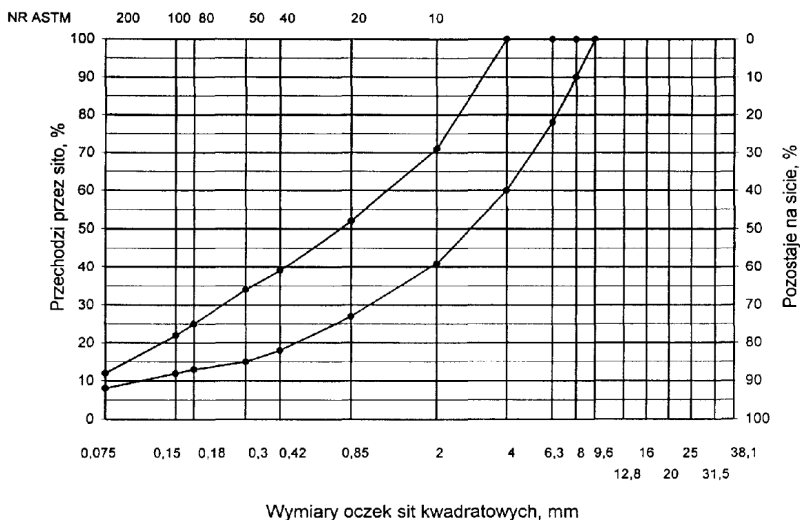
Rys. 3. Krzywe graniczne uziarnienia mieszanki mineralnej od 0 do 8mm, od 0 do 6,3 mm dla warstwy ścieralnej
